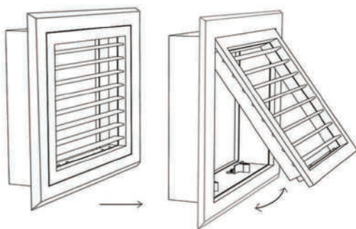
Cơ cấu tháo lắp chốt sập + bản lề
