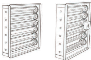
Cơ cấu điều chỉnh tay gạt, trục vít
